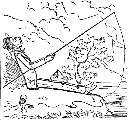
THE OBTUSE ANGLE.
